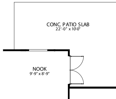
OPT. CONC. PATIO SLAB
